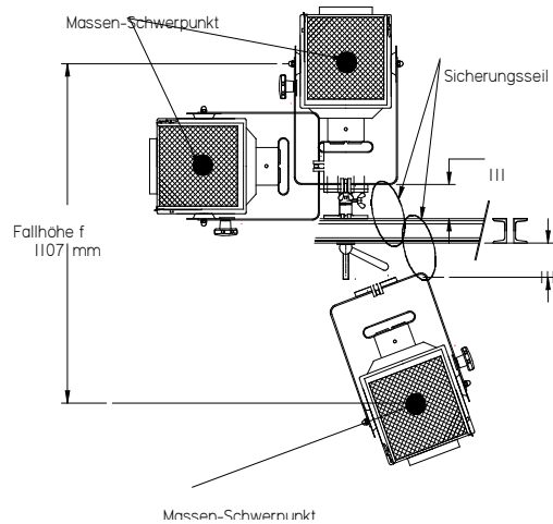
Abbildung 2 Fallweg beim stehenden Scheinwerfer, ca. 1,1 m
