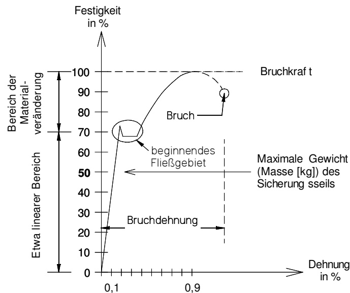
Abbildung 7 Schematische Darstellung des Spannungs-Dehnungs Diagramms
