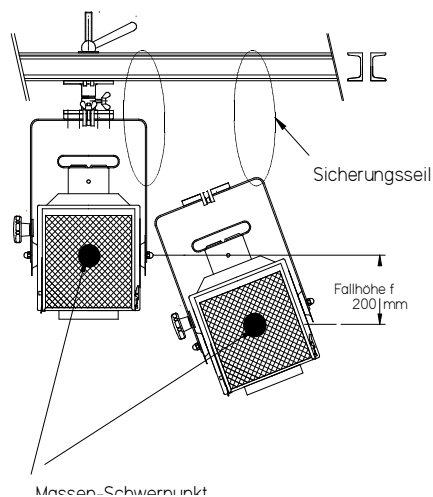
Abbildung 1 Fallweg beim hängenden Scheinwerfer - maximal 0,2 m
