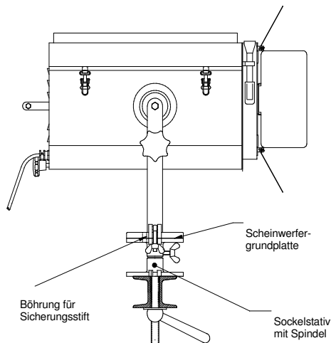
Abbildung 3 Bohrungen für Sicherungsstift Bei Verwendung des Sicherungsstifts kann der Scheinwerfer nicht mehr genügend kippen um herabfallen zu können. Es gibt keinen Fallweg
